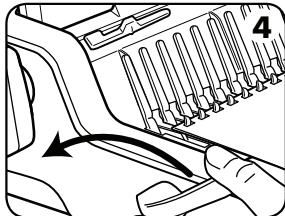
4. לאחר שכל הגליונות המנוקבים הוטענו על הספירלה, יש לדחוף את ידידת הספירלה אחורה עד הסוף כדי לסגור את הספירלה - ואז אפשר להוציא מהמכשיר את המסמך הכרוך.
